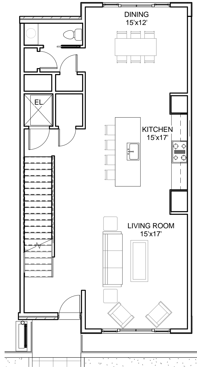
2 LEVEL 1 A-6 SCALE: 1/8" = 1'-0"
