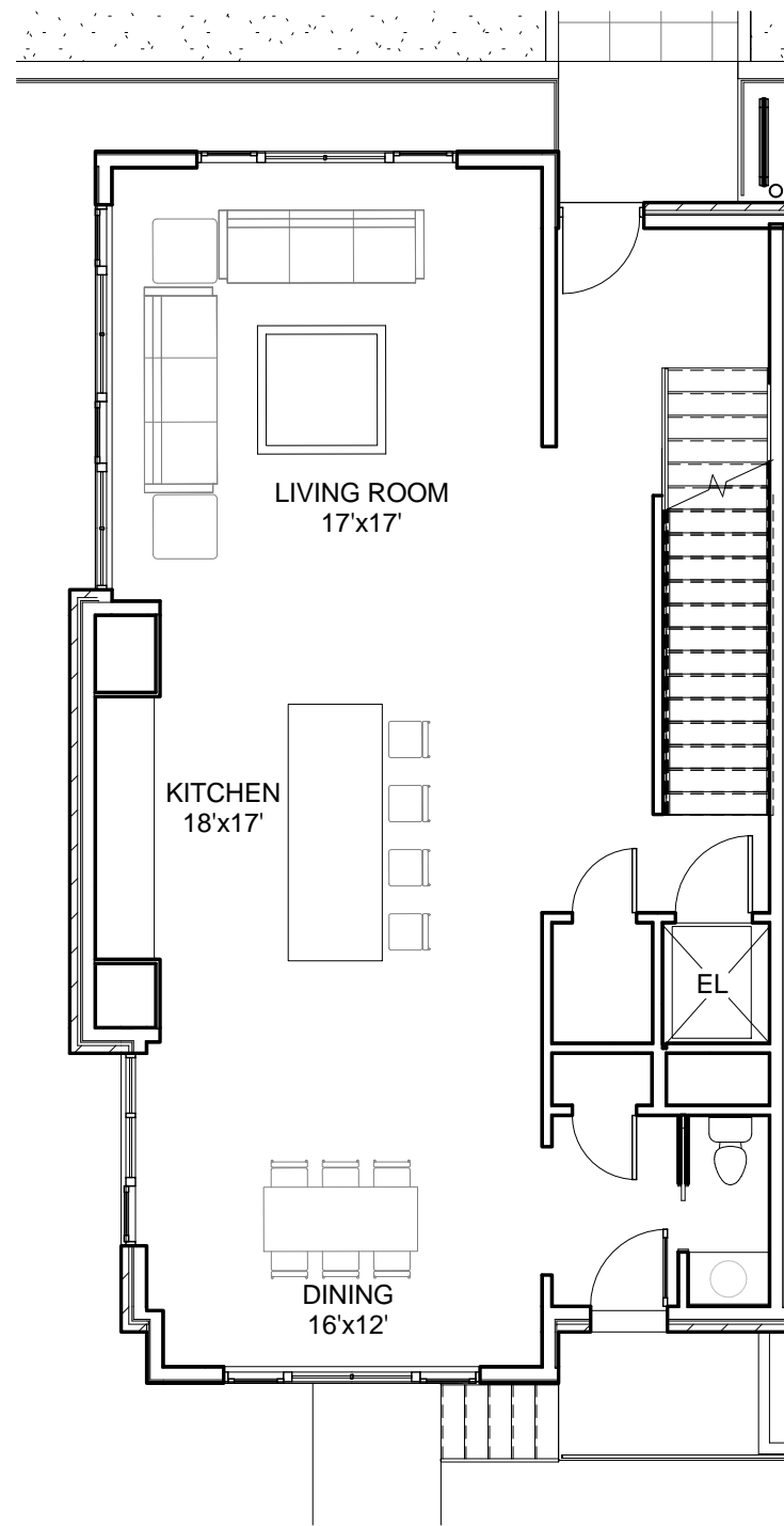
2 LEVEL 1 A-10 SCALE: 1/8" = 1'-0"
